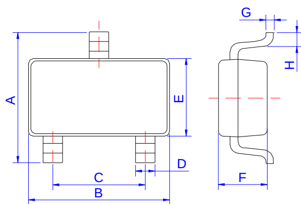
SOT-23-3L
